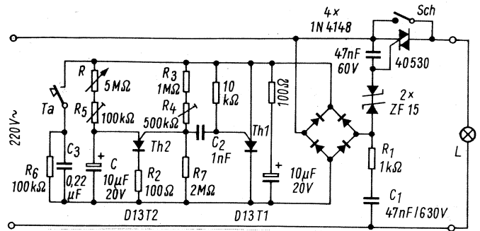
Bild 5. Zeitschalter mit selbsttätiger Entladung des zeitbestimmenden Kondensators; R kann bis 40 MΩ betragen
