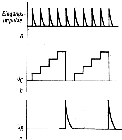
Bild 8. Verlauf der Spannungen in der Schaltung Bild 7
