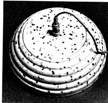
Bild 3. Sehr einfache und billige Behelfslösung, eine Blumenschale aus Schaumstoff dient als Reflektor für das Mikrofon; a = Vorderseite, b = Rückseite, die Kabelkupplung dient als Befestigung. Aufnahme: O. Limann
