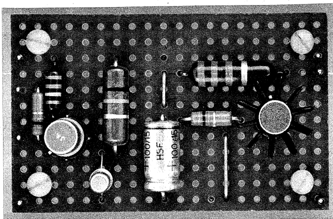
Unten: Bild 2. Aufbau des kontaktlosen Thermostaten. Links: Platine des Mustergerätes; rechts: Bestückungsplan (siehe auch Stückliste)
