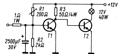
Schaltung einer einfachen Lichtrhythmusanlage
