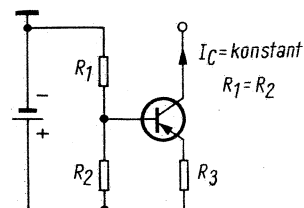
Bild 3. Einfache Konstantstromquelle mit Transistor
