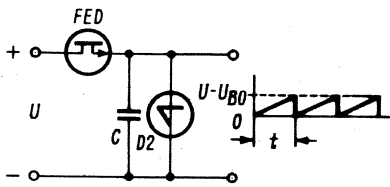
Bild 4. Sägezahn-generator mit FE-Diode und Vierschichtdiode
