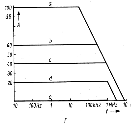
Bild 8. Mit Hilfe der Gegenkopplung läßt sich das Übertragungsverhalten eines Operationsverstärkers dem Verwendungszweck anpassen. Ohne Gegenkopplung beträgt die Leerlaufverstärkung 100 dB (a). Ein Spannungsteiler im Gegenkopplungsweig läßt in der Schaltung (b) die Verstärkung auf 60 dB absinken (b), während eine Änderung des Spannungsteilerverhältnisses eine Abnahme der Verstärkung auf 40 dB zur Folge hat (c). Soll die Verstärkung noch weiter herabgesetzt werden, so werden in den Gegenkopplungskreisen Blindwiderstände notwendig. Im Fall (d) beträgt die Verstärkung noch 20 dB, während sie für die Schaltung (e) auf 0 dB zusammenbricht. Im Diagramm (f) ist der Einfluß der verschiedenen Gegenkopplungsschaltungen auf die Verstärkung und auf den Frequenzgang festgehalten
