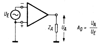
Bild 6. Die Verstärkung des Operationsverstärkers entspricht dem Quotienten von Ausgangsspannung zu Eingangsspannung. Die Eingangsspannung liegt zwischen den beiden Eingängen des Verstärkers
