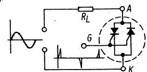
Bild 2. Ersatzweise Darstellung eines Triacs
