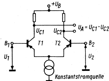
Bild 2. Prinzipschaltung eines Differenzverstärkers mit Konstantstromquelle
