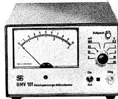
GMV 101 Gleichspannungs-Millivoltmeter
